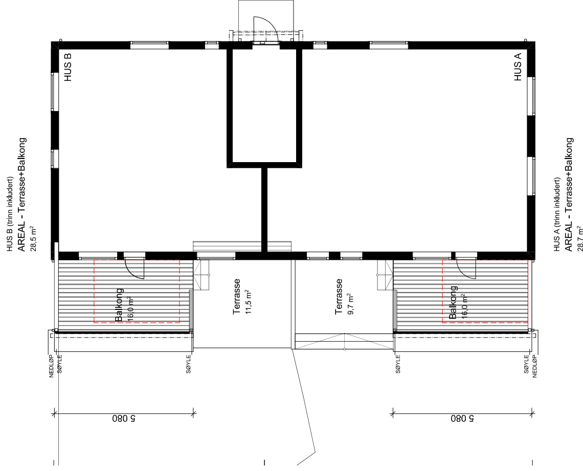
Plan 1.Etasje
