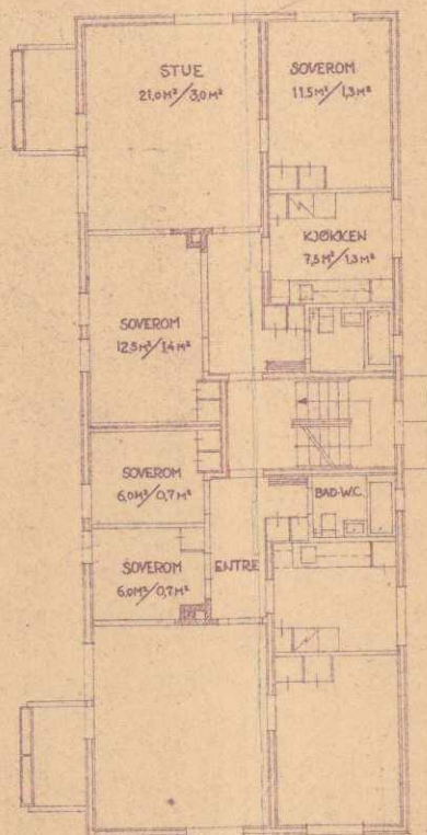
2. ETASJE
