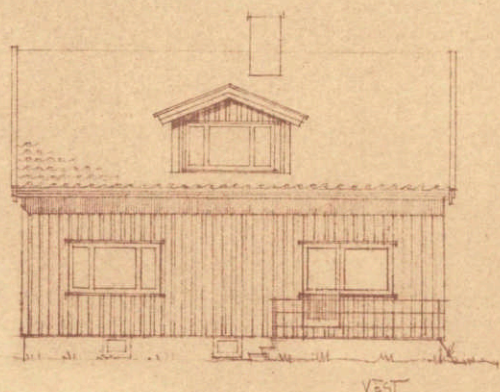
Vest
