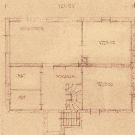
FÖRSTA PLAN.
