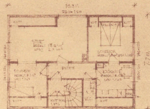
ANDRA PLAN.
