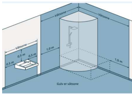
§ 13-16 Figur 1: Minste utstrekning på vannrett sjikt i våtrom.
